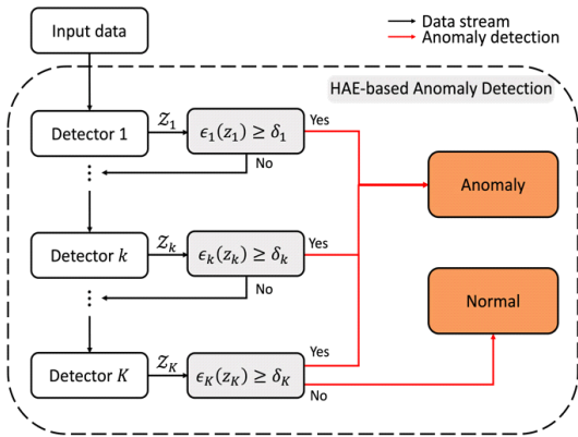
그림 1. HAE 기반 이상탐지 구조 Fig. 1. Structure of HAE-based anomaly detection
